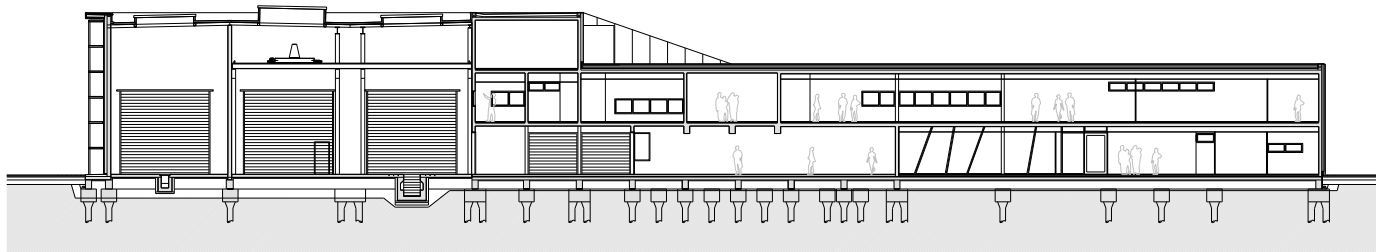
LONGITUDINAL SECTION
